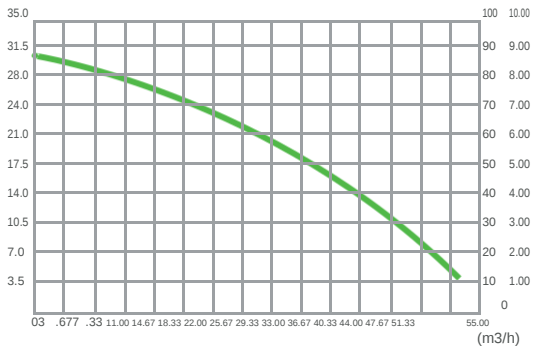
(M) Curva de rendimiento DS30 EFF(%) P1(W)
