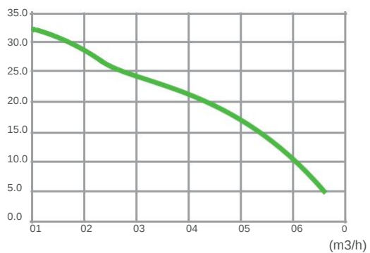
(M) Curva de rendimiento DDP80
