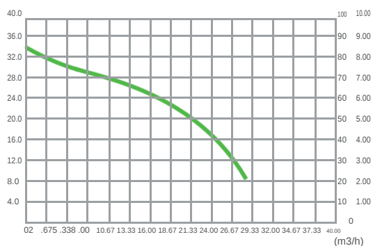
(M) Curva de rendimiento DS20 EFF(%) P1(W)
