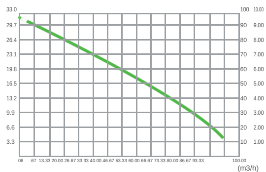
(M) Curva de rendimiento DS40 EFF(%) P1(W)
